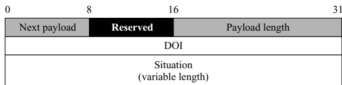
Figure 18.31 SA payload
