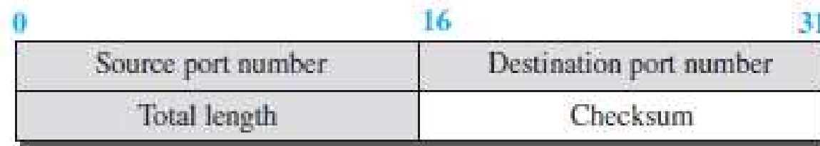
b. Header format
